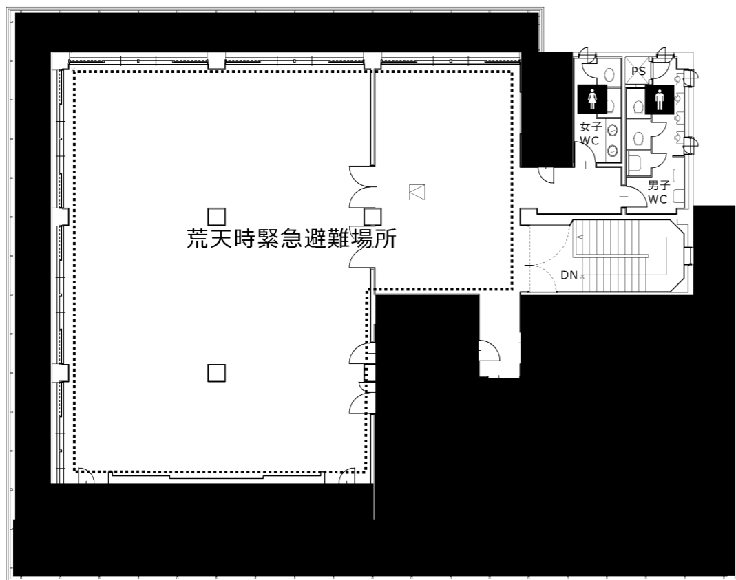
平岸庭球場管理事務所 3階平面図
